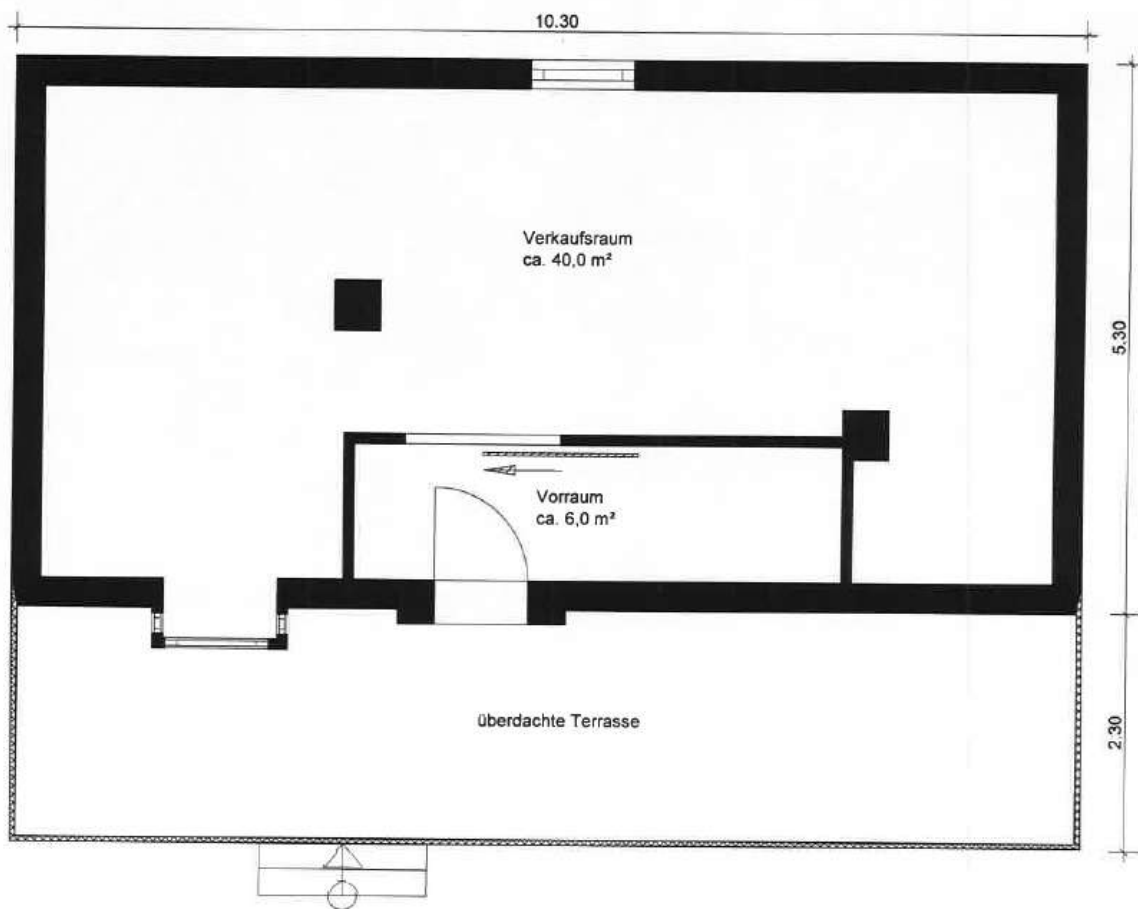
Grundrisskizze Erdgeschoss - Platz der Jugend 2, Brachwitz -
